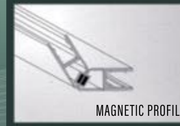
DM-092 | 135° 8mm (2.2mtr.) 10mm (2.2mtr.) 10mm (2.5mtr.) 12mm (2.2mtr.)
